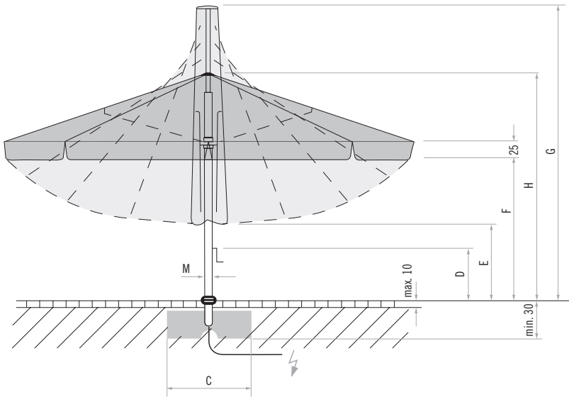
Loser Deckbelag max. 10 cm, Betondicke min. 30 cm (Frosttiefe beachten), Wasserabfluss, 1. Zuleitung elektrisch.
